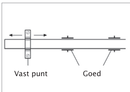
figuur A Bevestiging van buizen: rechte buis, slechts één bevestigingspunt: goed
